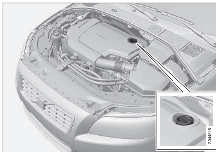
Заправочная горловина 8
