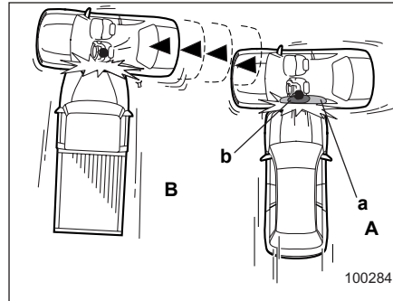
A) Первый удар B) Второй удар a) Подушка-шторка b) Боковая подушка безопасности
