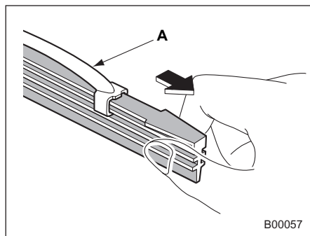
А) Металлический держатель
