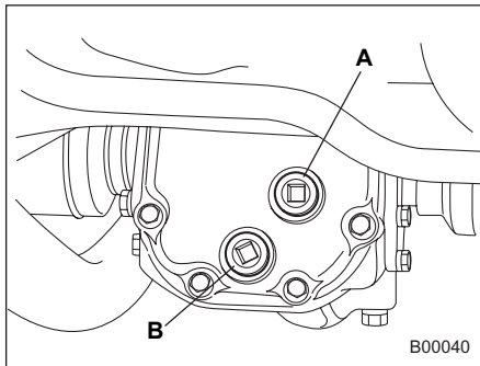
Модели с двигателем объемом 2,5 л; 2,0 л с МКПП; 3,0 л с МКПП
