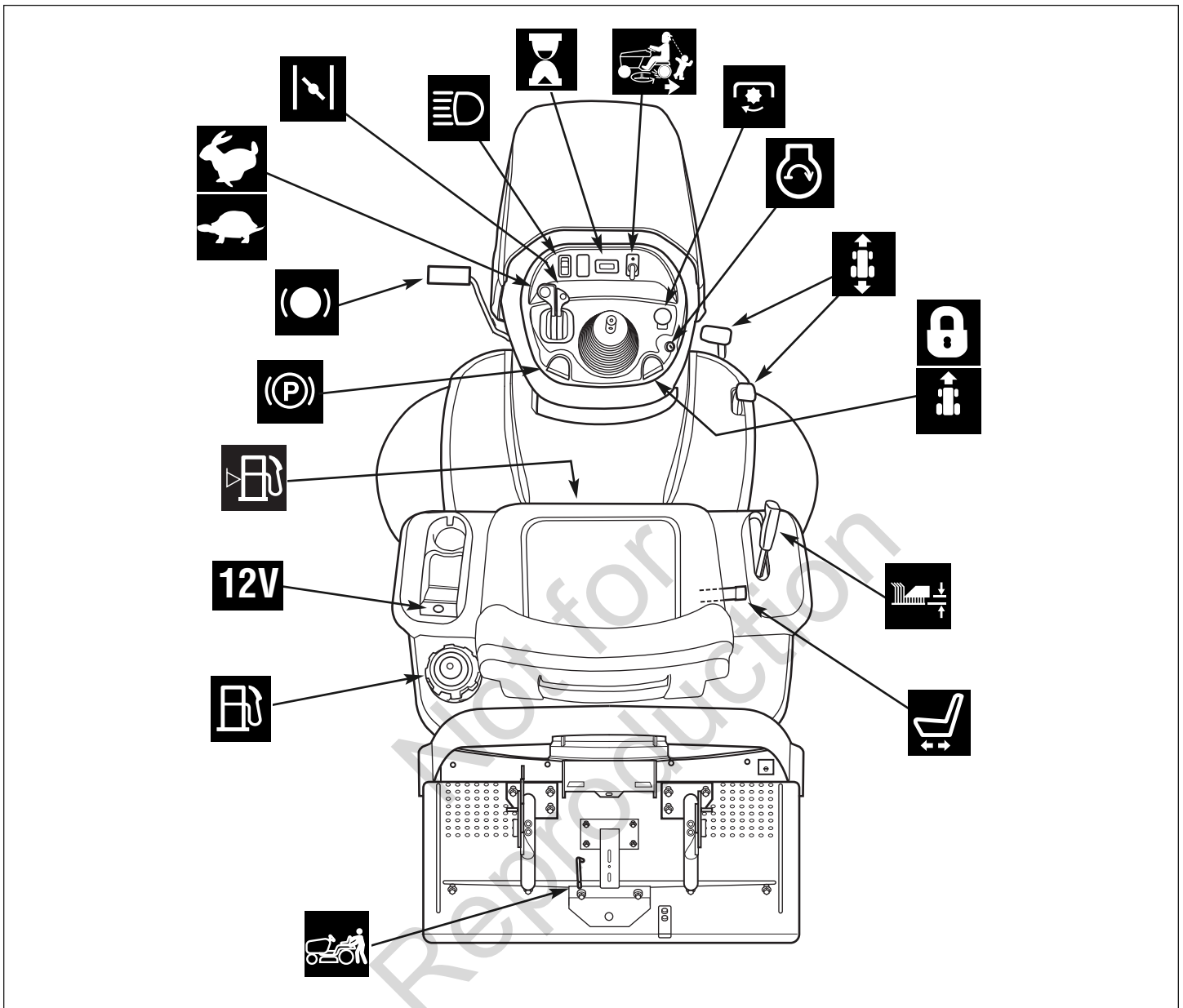
Ovladače traktoru
