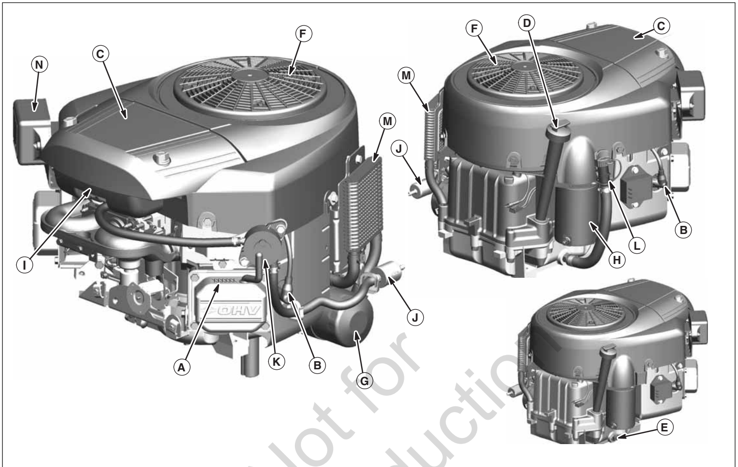
Motorbedieningselementen
