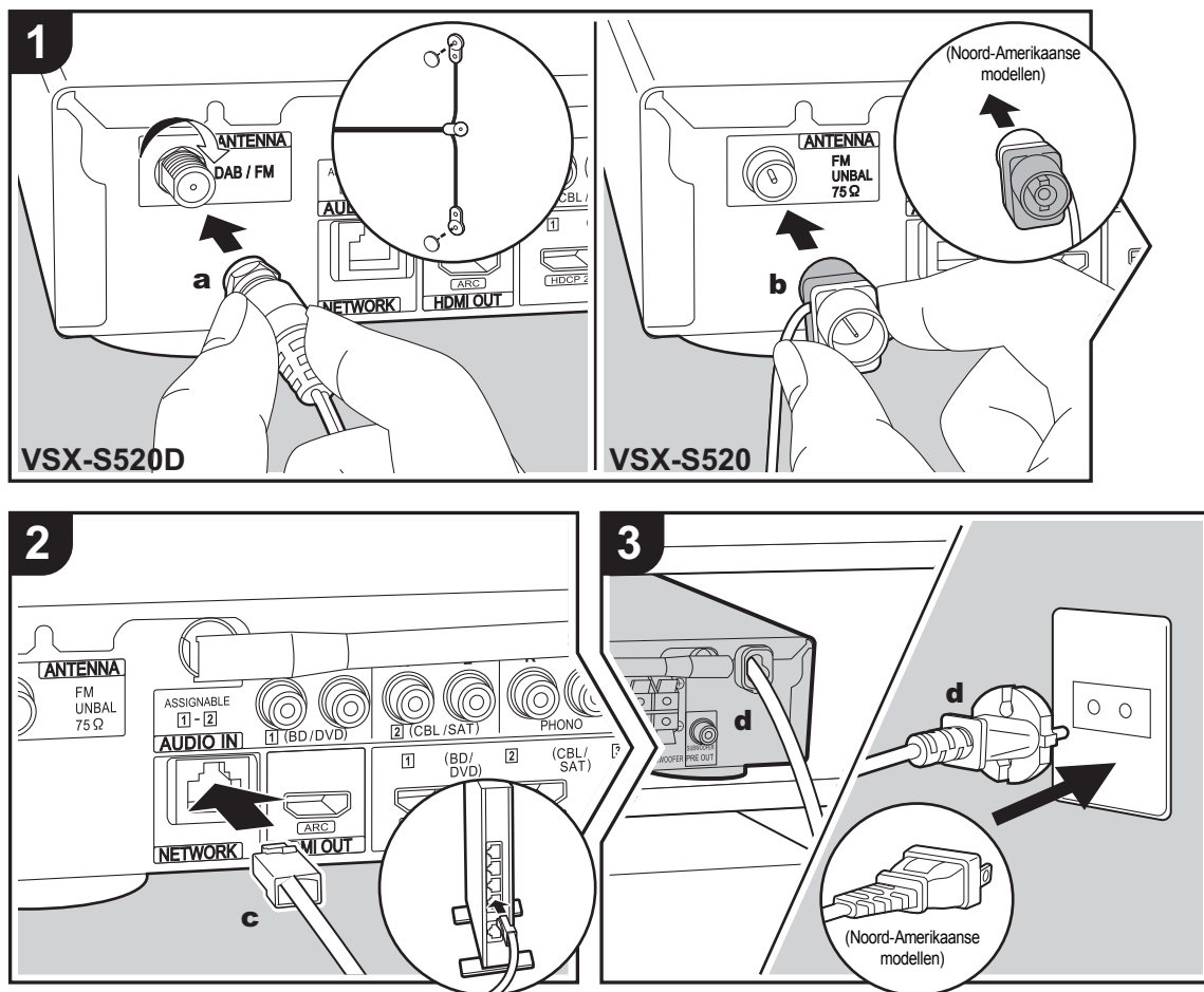
a DAB/FM-antenne, b FM-binnenantenne, c Ethernet-kabel, d Netsnoer
