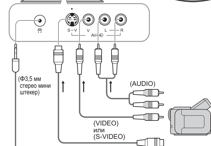
Видеокамера / Игровая приставка
