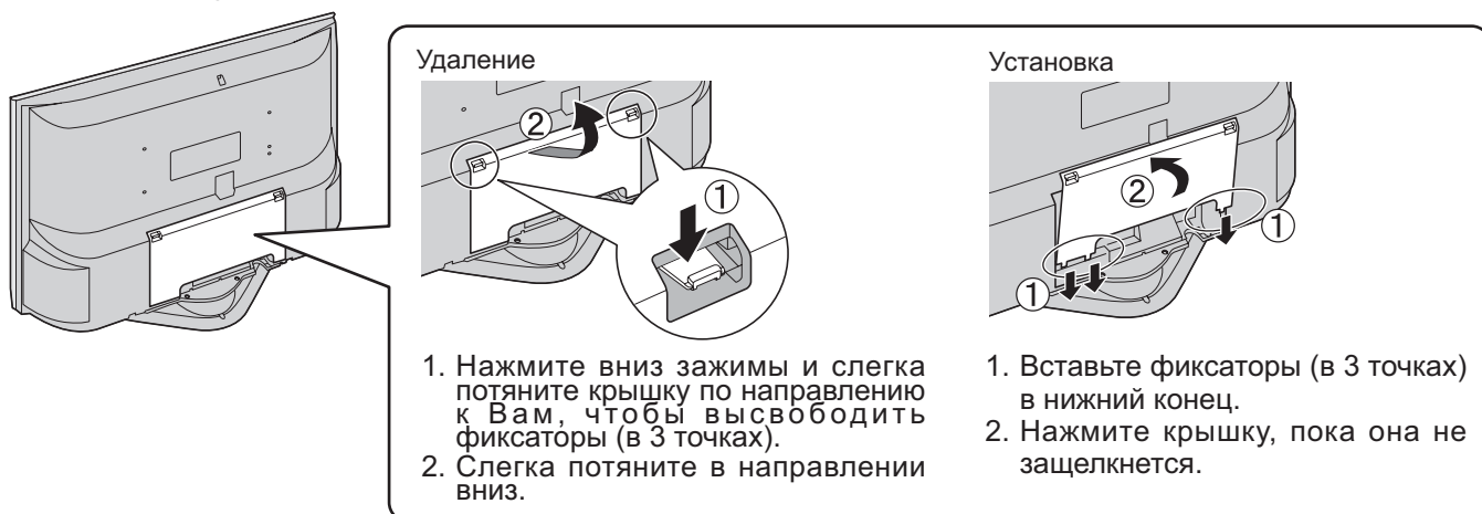
Задняя панель телевизора
