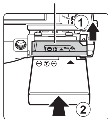
Батарейный отсек
