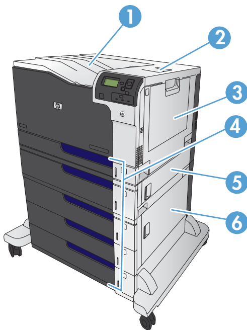
Рисунок 11-1 Места замятий
