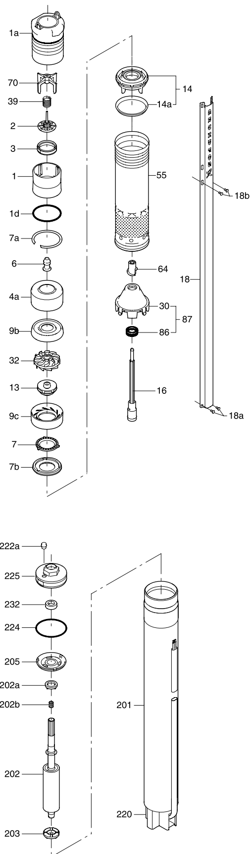
Рис. 34. Спецификация материалов компонентов насоса типа SQ.
