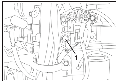
1. Отверстие для подключения измерителя давления (правый борт)
